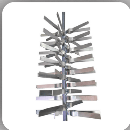
فیکسچر انگشتی صفحه ای
